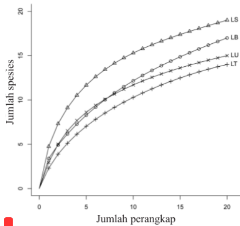
Gambar 2. Kurva akumulasi spesies semut yang ditemukan pada empat daerah penelitian. LS: Desa Negara Ratu, Lampung Selatan; LB: Desa Sekincau, Lampung Barat; LU: Desa Cahaya Negeri, Lampung Utara; LT: Desa Sukadana Baru, Lampung Timur. Proporsi spesies hasil observasi/estimasi Chao: LB = 17/33 (52%); LS = 19/28 (68%); LT = 14/17 (85%); dan LU = 15/21 (71%).
