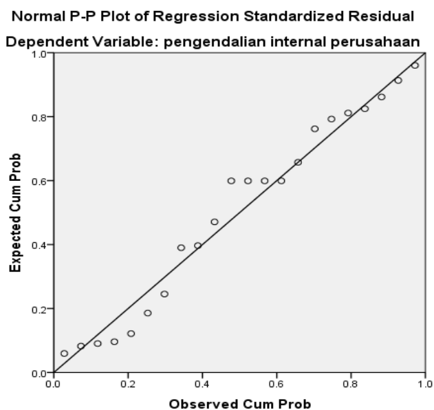
Gambar 4.1 Uji Normalitas
